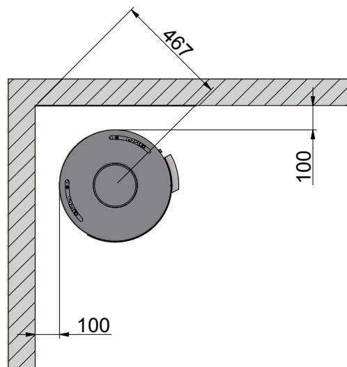
Installation en angle à 45°
