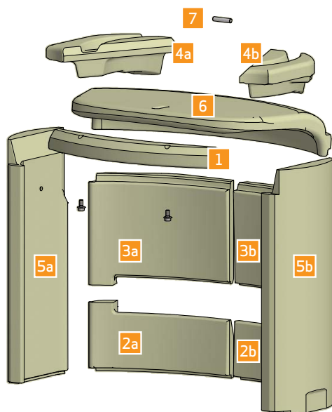
Monter les plaques de vermiculite 2a et 2b
