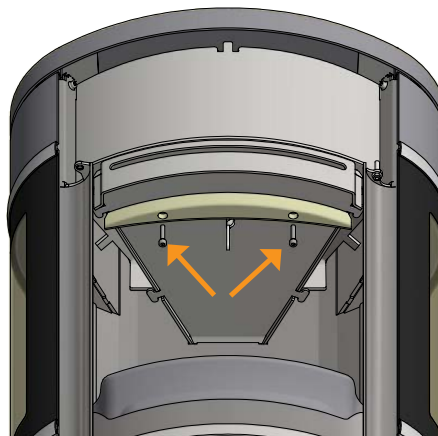
Monter la plaque de Vermiculite 1 avec 2 vis
