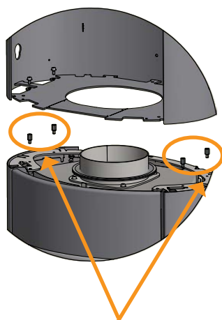
Douille entretoise
