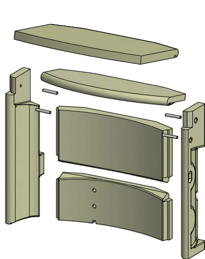
65-2, 65-4, 65-8 et 65-10 (avec vitres latérales)
