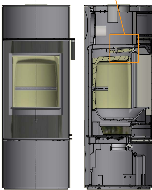
Déflecteur de fumée supérieur
