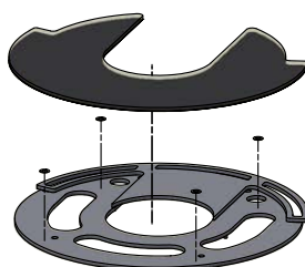
Plaque supérieure de verre pour sortie par le haut
