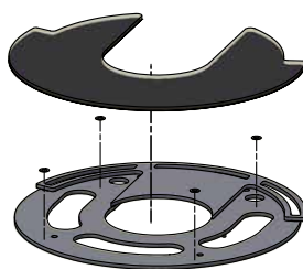
Plaque supérieure de verre pour sortie par le haut
