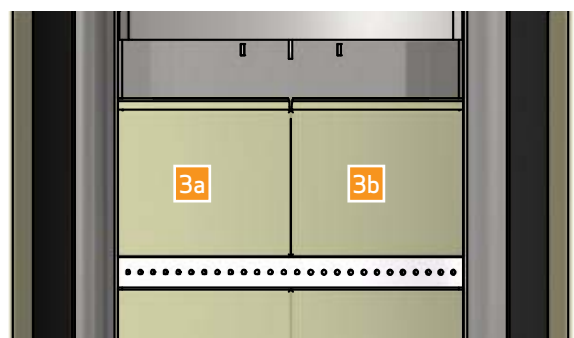
Monter les plaques de vermiculite 3a et 3b
