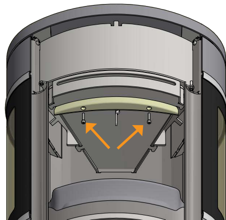
Monter la plaque de Vermiculite 1 avec 2 vis
