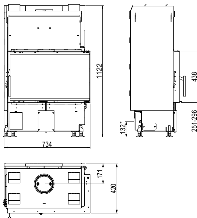
Croquis Scan 5107 avec bouclier thermique du côté de la cloison pare-feu (accessoire)
