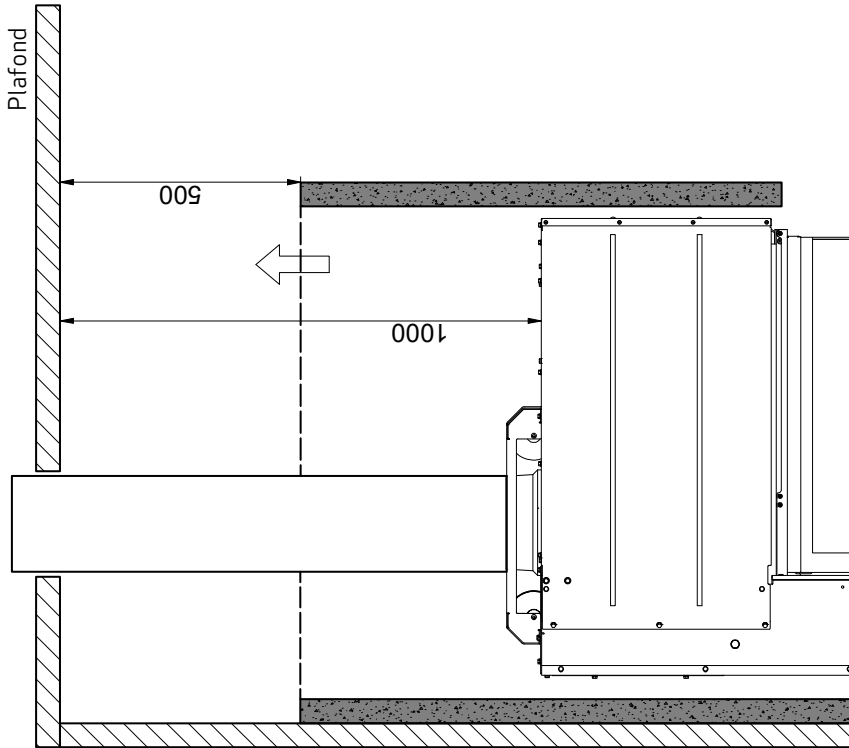
Configuration avec conduit d'évacuation des fumées vertical isolé - ouverture de convection
