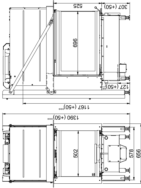
Scan 5005 avec construction de soutien*
